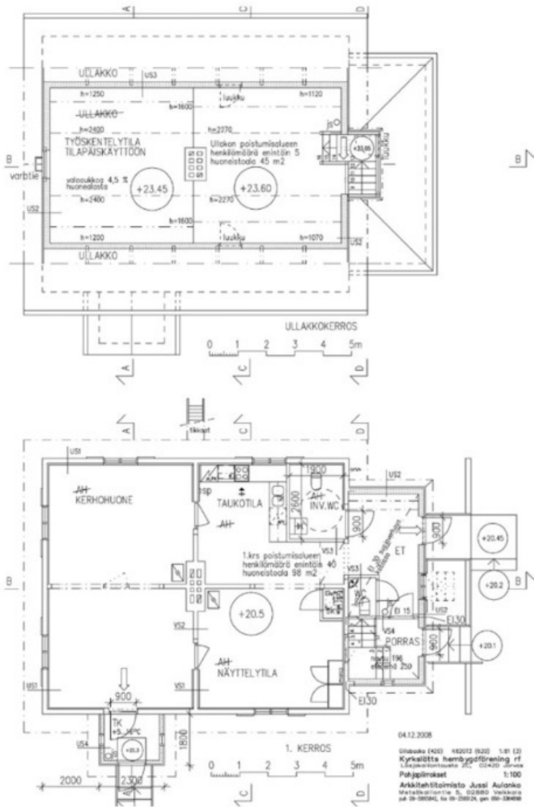
I bottenvåningen på 116 kvm finns mötes- och seminarierum, övre våningen reserveras för arbets- och förvaringsutrymmen. Ritning: Jussi Aulanko
